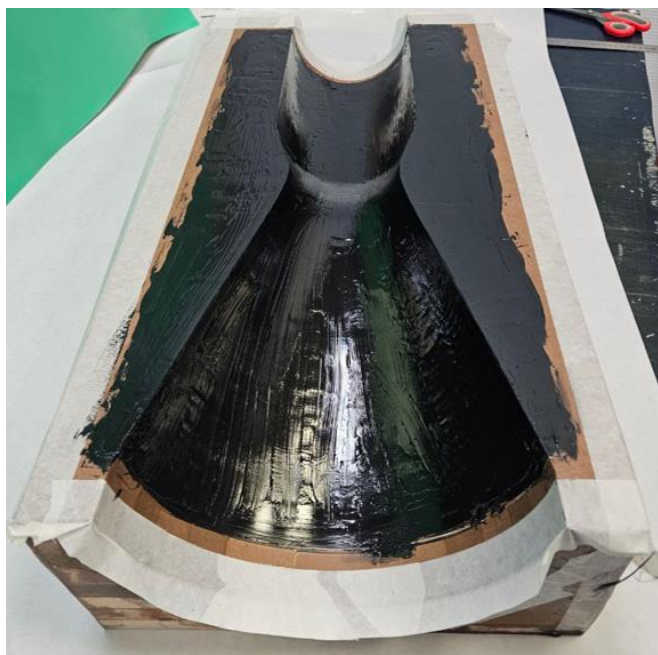
Рисунок 2– Пример готовой оснастки с использованием гелькоута CP200C
